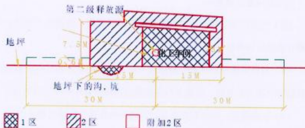
附图 1.4-1 生产车间爆炸危险区域图
