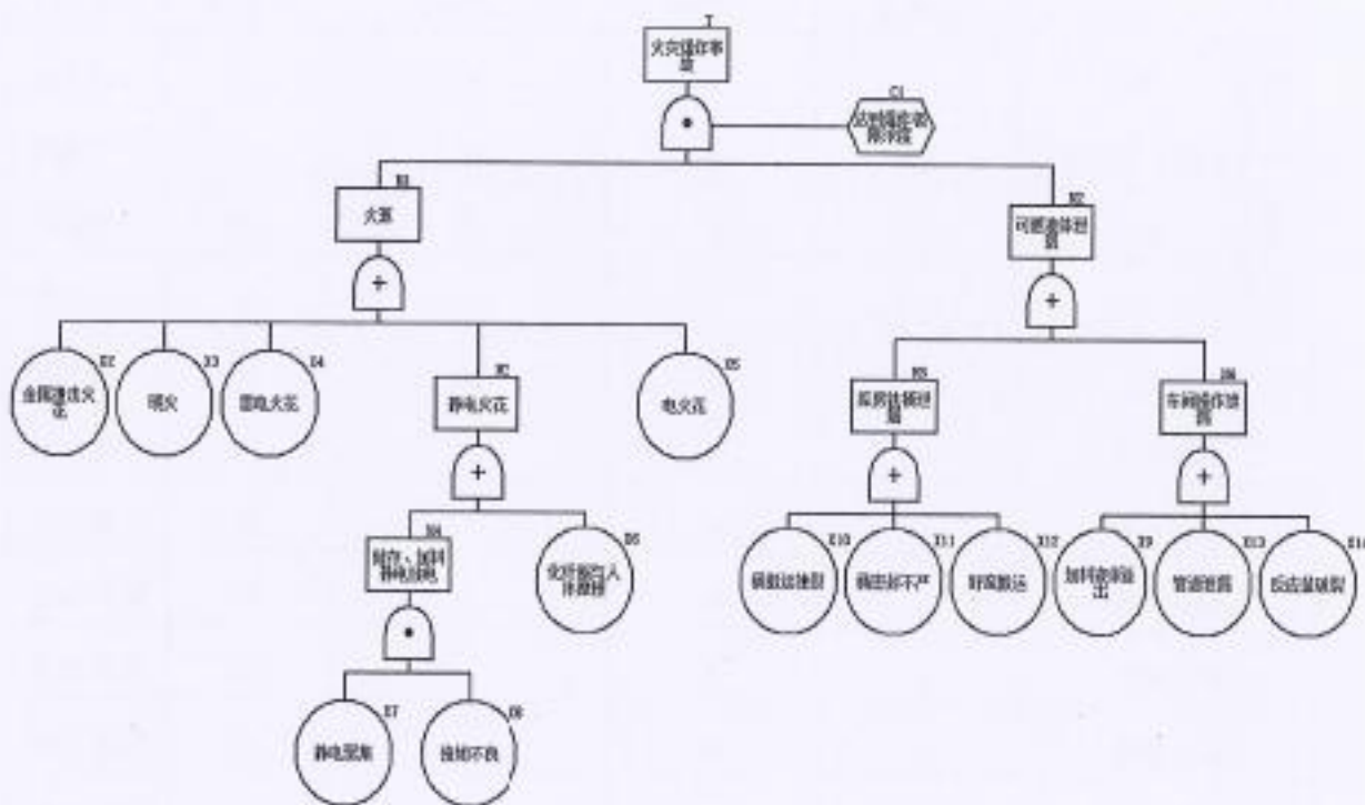
附图 2.6-1 火灾爆炸事故树分析图
