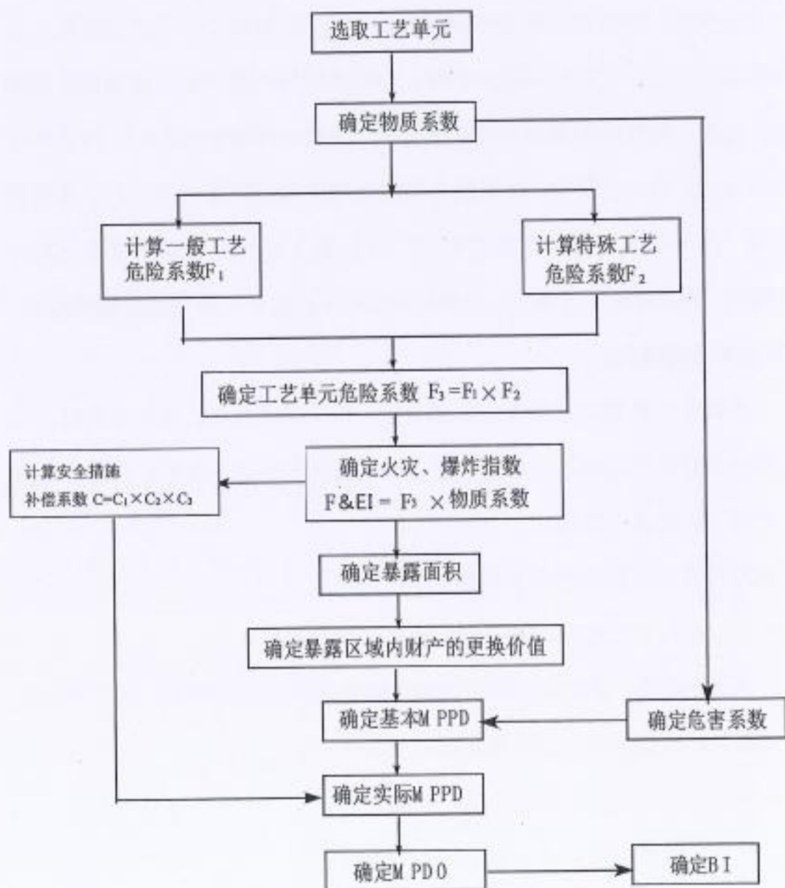
附图 5.2-1 道化学火灾爆炸危险指数法评价程序图
