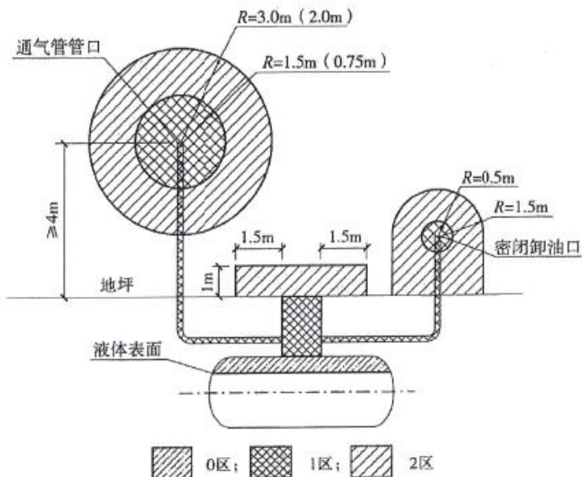
图 3-3 汽油埋地卧式储罐爆炸危险区域划分
