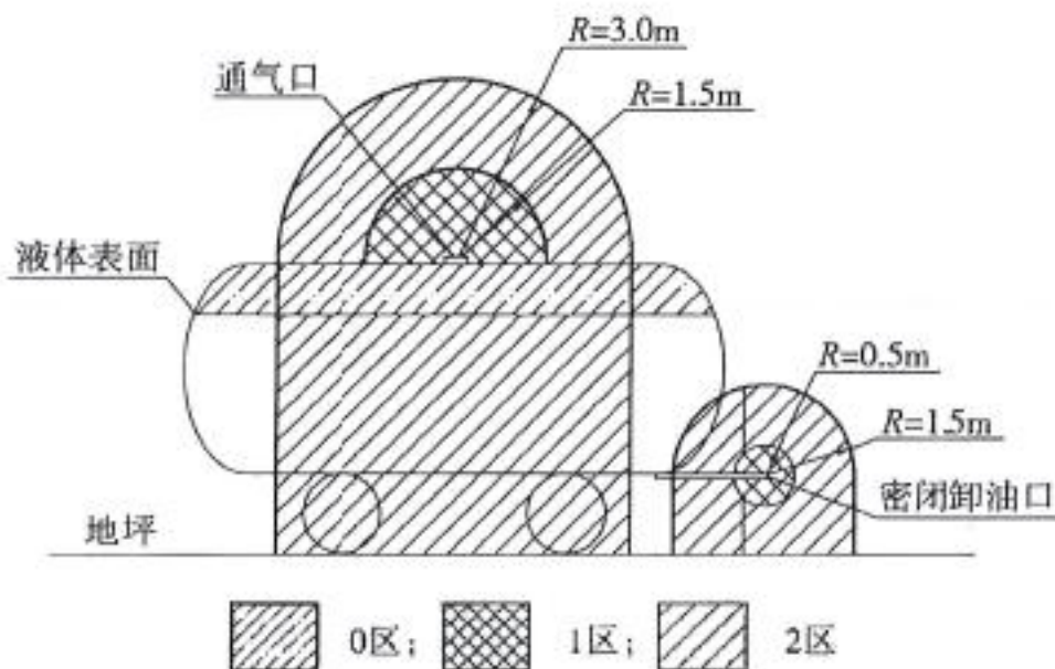
图 3-2 汽油油罐车卸汽油时爆炸危险区域划分
