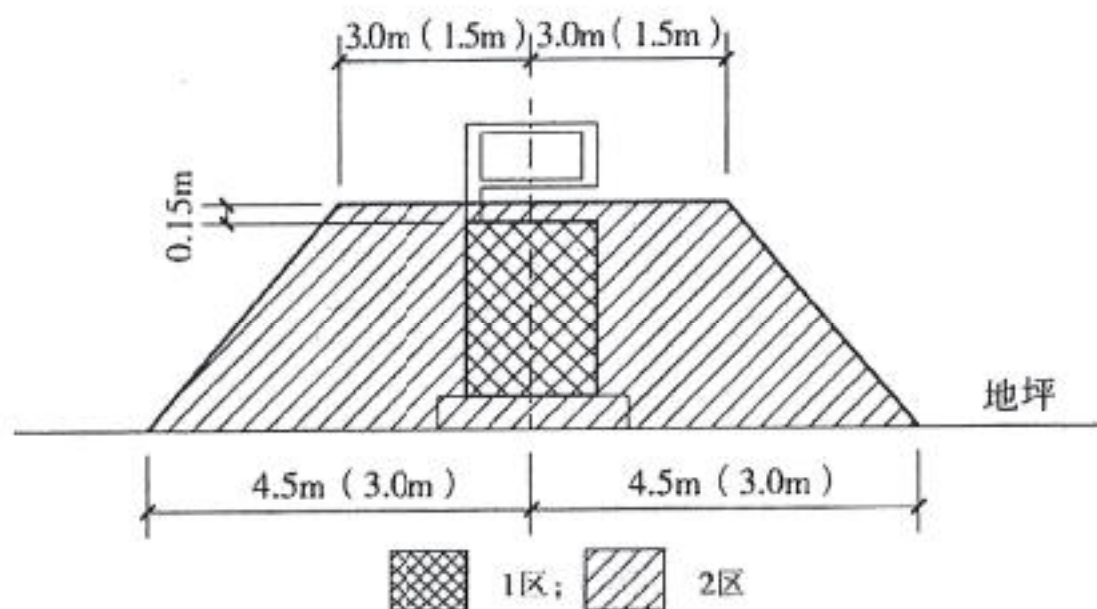
图 3-1 汽油加油机爆炸危险区域划分
