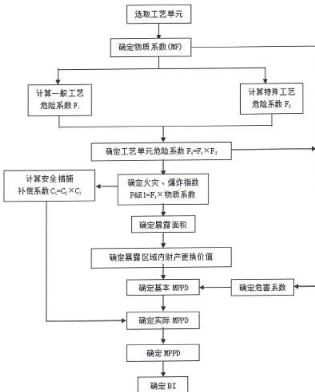
图 4-1 道化学火灾、爆炸危险指数评价法（第七版）评价程序
